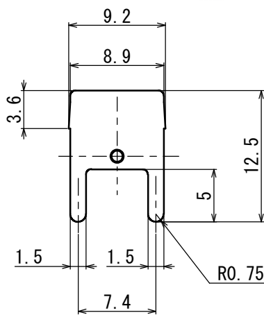
セット寸法例 Example of dimension for SET
