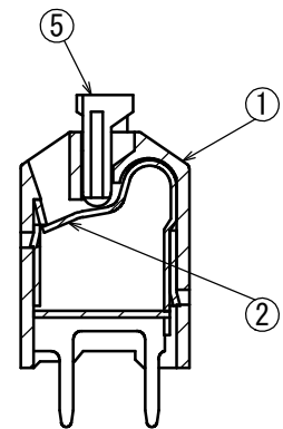
断面図C(2 / 1)
