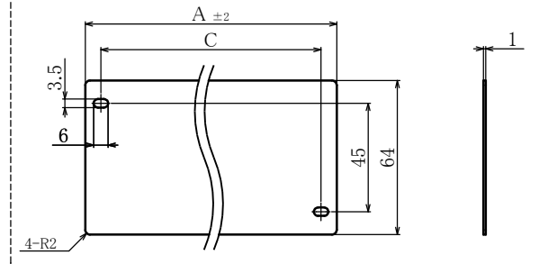
断面図 E-E
