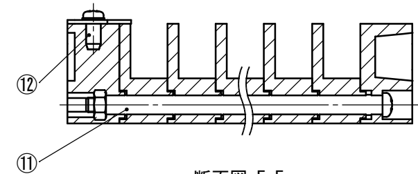
断面図 E-E
