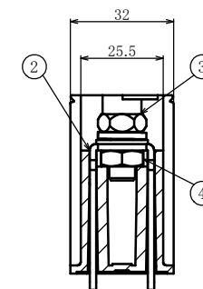
断面図A(1 / 1.5)
